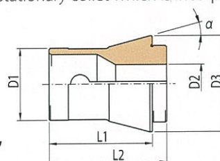
割り入れブランク Slotted blank
