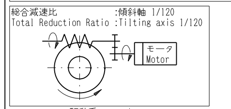
駆動系スケルトン Skelton Drawing of Drive System
